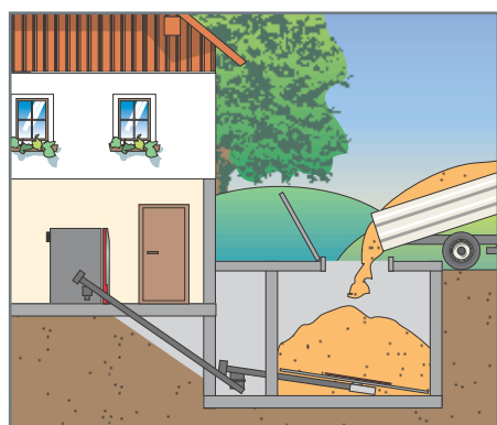
Silo enterré avec vis de remonter vers la chaudière située au RdC.
