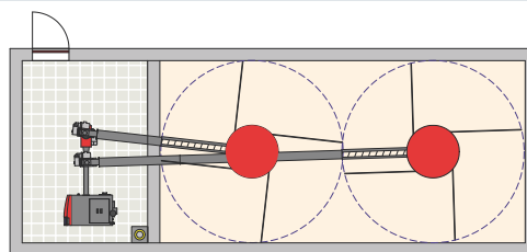
Tube de chute avec bride haute supplémentaire pour raccordement sur raccord double en Y
